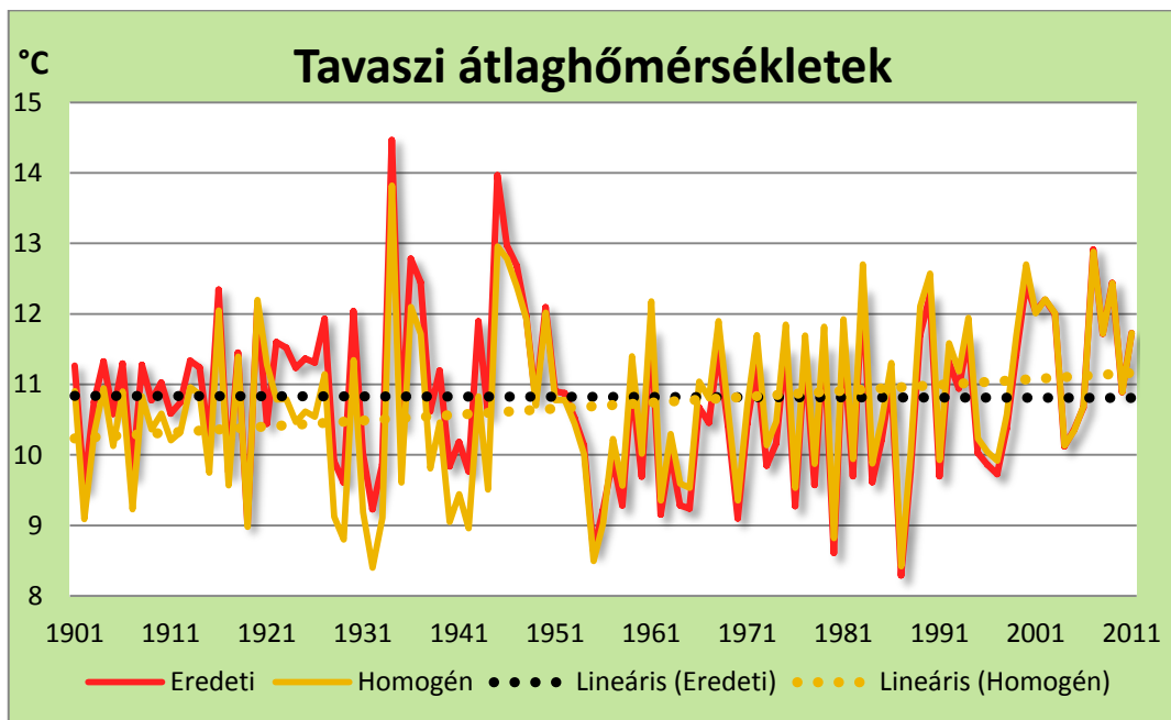
19. ábra Eredeti és homogén adatsorok tavaszi középhőmérsékletei Pécssett
