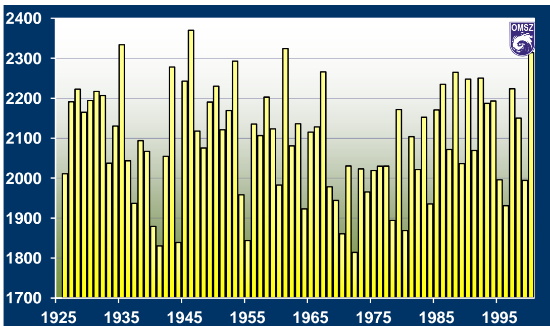
17. ábra A napfénytartam évi összege Pécsen a XX. században
