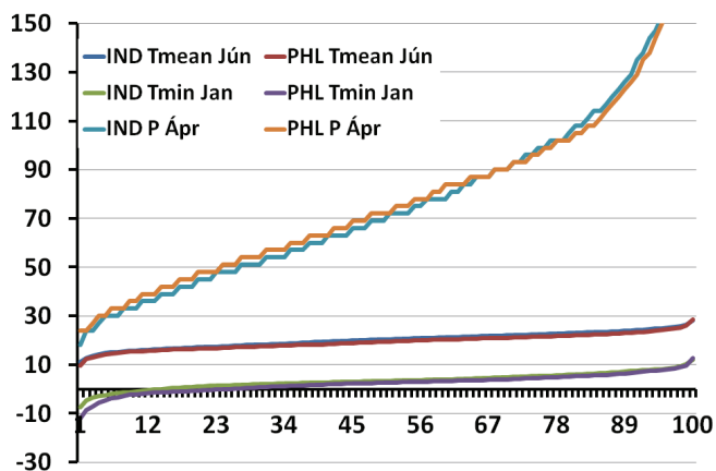
5. ábra: Három éghajlati paraméter (júniusi középhőmérséklet, januári minimum-hőmérséklet, áprilisi csapadékösszeg) eloszlásfüggvénye a lepkeszünnyogok (PHL) és indikátoraik (IND) esetén
