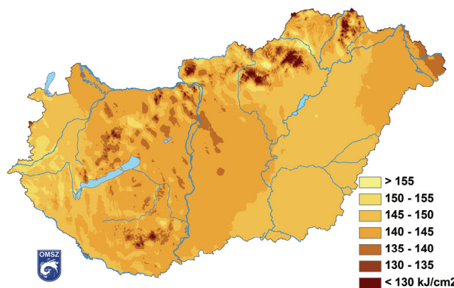
3. ábra: A tavasz globálisugárzás összege (kJ/cm²)
