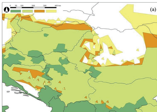
4. ábra: A lepkészünnyogokra (a) és az indikátor növényfajokra (b) készült modelleredmények kárpát-medencei kivágatának összevetése
