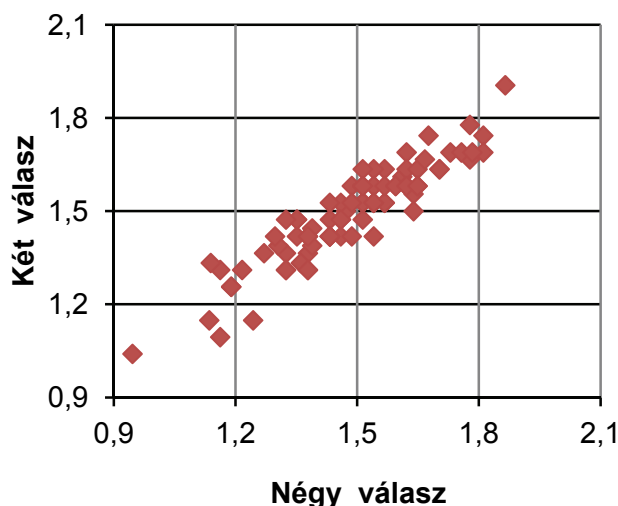
1. ábra: A négy választeszt és annak két válaszosra redukált változata alapján adható egyéni frontérzékenységek kapcsolata. A redukció során az eredeti 0 vagy 1 pontnak megfelelő értékeket 0,5-tel, a 2 és 3 pontot 2,5-tel helyettesítettük. (A két változó korrelációja 0,922.).
