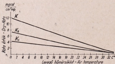
1. ábra — Fig. 1.: A katatermométer teljes ( K ), konvekciós ( K_k ) és sugárzásos ( K_s ) hőleadása nyugvó levegőben. — Heat losses of the catathermometer: K total heat loss, K_k losses by convection, K_s losses by radiation.
