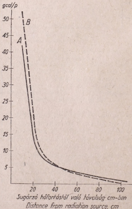
3. ábra — Fig. 3.: A katatermómeter által felvett sugárzó hőmennyiség a hőforrástól mért távolság szerint: A = 1,1-1,35 m/mp légáramlás, B = nyugvó levegő. — Heat absorption by the catathermometer as a function of the distance from the radiating source. A : air movement of 1,1-1,35 m/s, B : still air.
